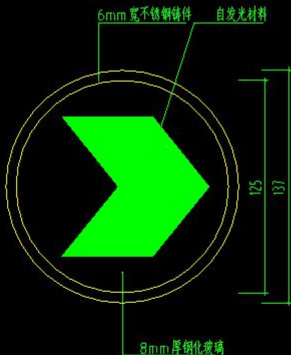
5 地面疏散指示放大图
