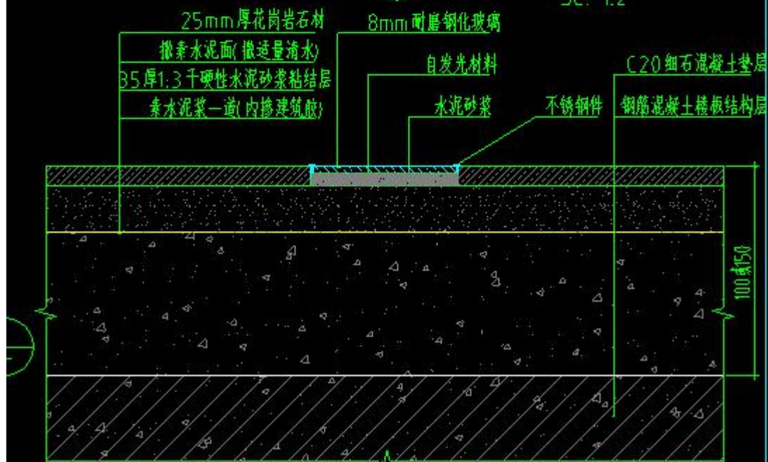
4 自发光疏散标识设置定位剖面大样
